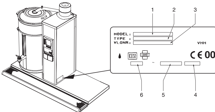
Abb. 1 Typenschild
